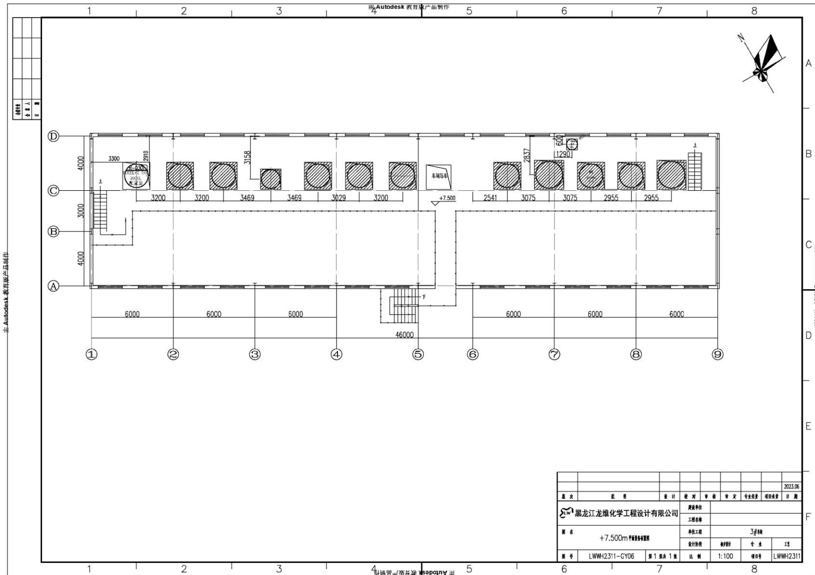
附图 7 设备平面布置图三
